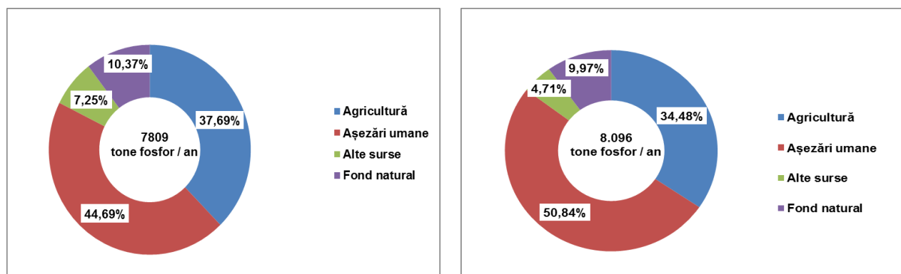
Figura 2.2.3.4. Rezultatele aplicării scenariului de bază pentru sursele de emisii ale fosforului (punctiforme și difuze) în anul 2012 (stânga) și anul 2021 (dreapta)
