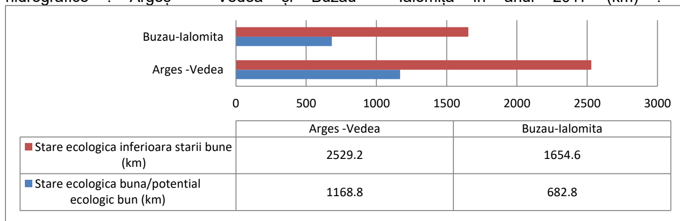
Figura 2.2.1.1.2. Starea ecologică/potențialul ecologic al cursurilor de apă monitorizate (corpuri de apă naturale, puternic modificate, artificiale - râuri) pe spații/bazine hidrografice în anul 2017 (km) (Sursa : Administrația Națională "Apele Române")
