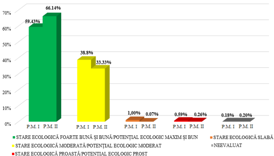
Figura 2.2.3.5. Evoluția stării ecologice/potențialului ecologic al corpurilor de apă de suprafață –cel de al 2-lea Plan de Management (2021) și primul Plan de Management (2015) (Sursa datelor: Administrația Națională „Apele Române”, Planul Național de Management actualizat aprobat prin HG nr. 859/2016 pentru aprobarea Planului Național de management actualizat aferent porțiunii din bazinul hidrografic internațional al fluviului Dunărea care este cuprinsă în teritoriul României)
