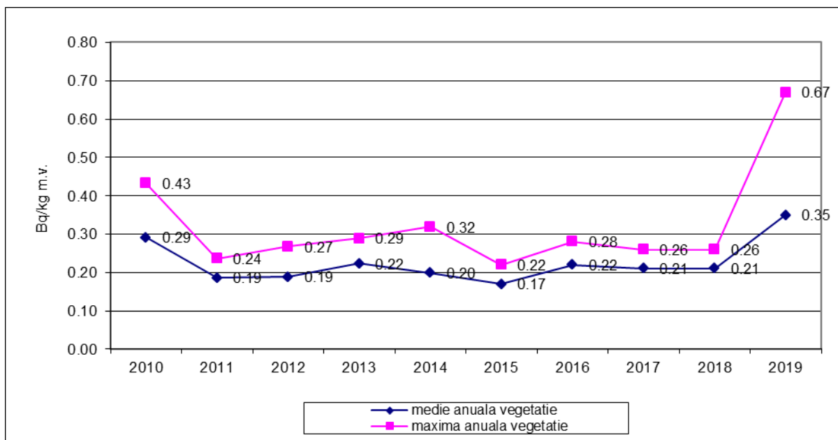
Figura nr. IX.1.4.1. Variația mediilor și maximelor anuale ale activității beta globale a vegetației spontane în municipiul Călărași, în perioada 2010 – 2019
