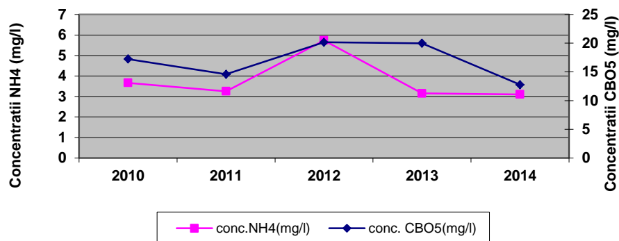
Figura 2.2.1.1.6. Evoluția indicatorilor CBO 5 și NH 4 + în cursurile de apă din județul Călărași, în perioada 2010-2014; (Sursa : Administrația Bazinală de Apă Argeș – Vedea)
